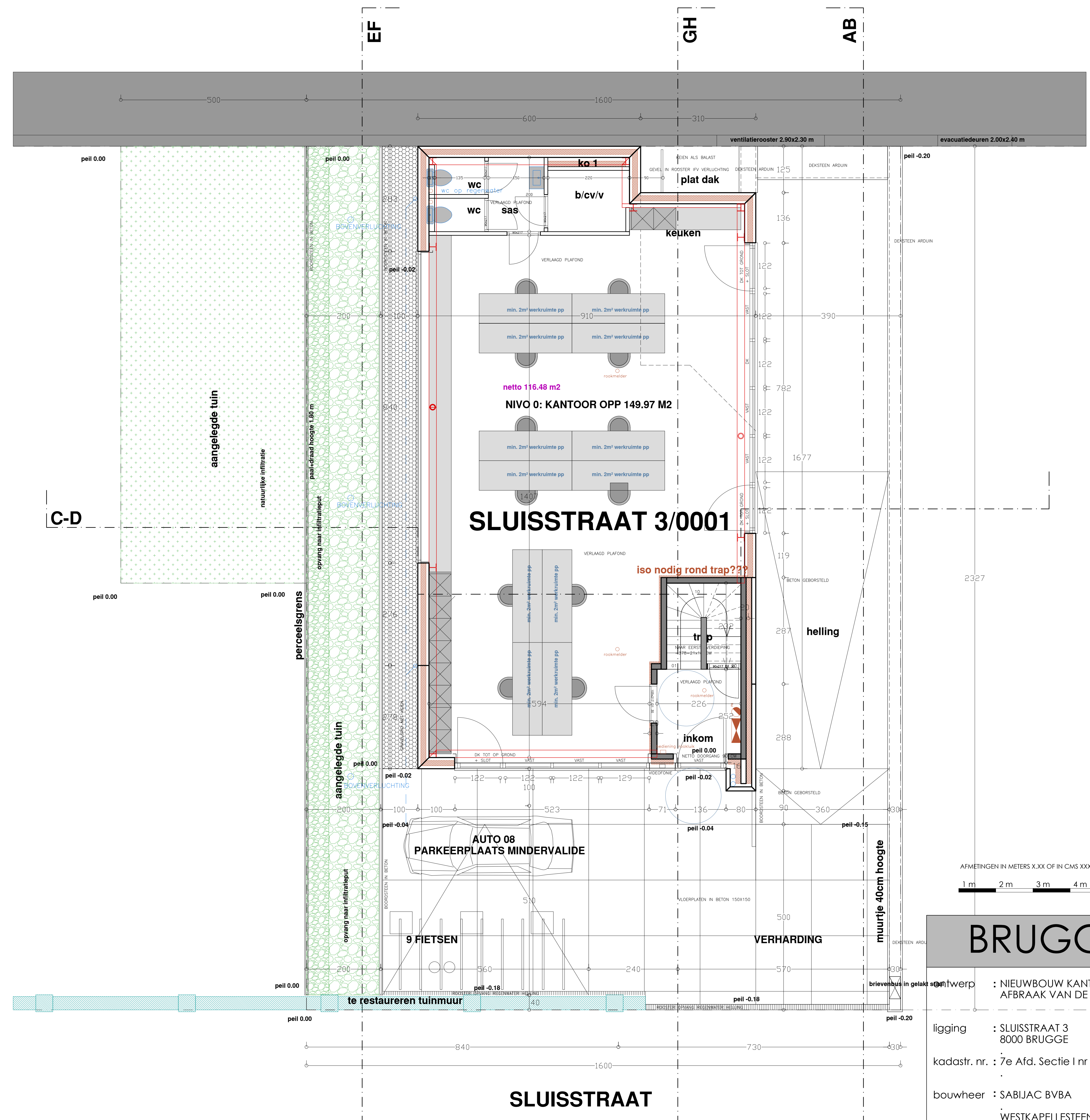
GELIJKVLOERS
